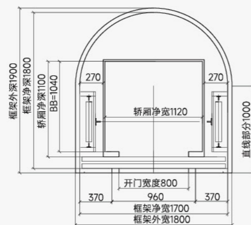
方形轿厢
