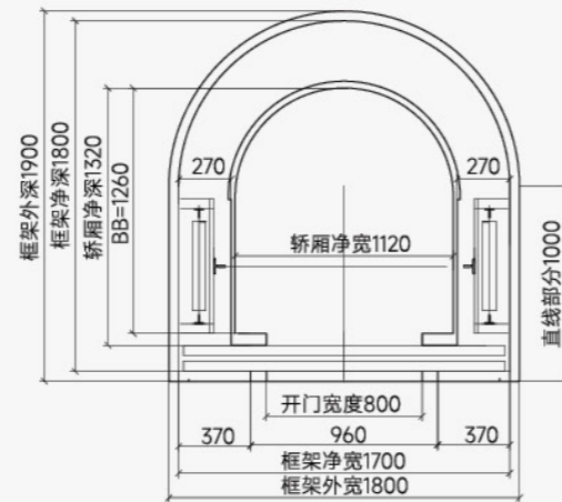
半圆形轿厢
